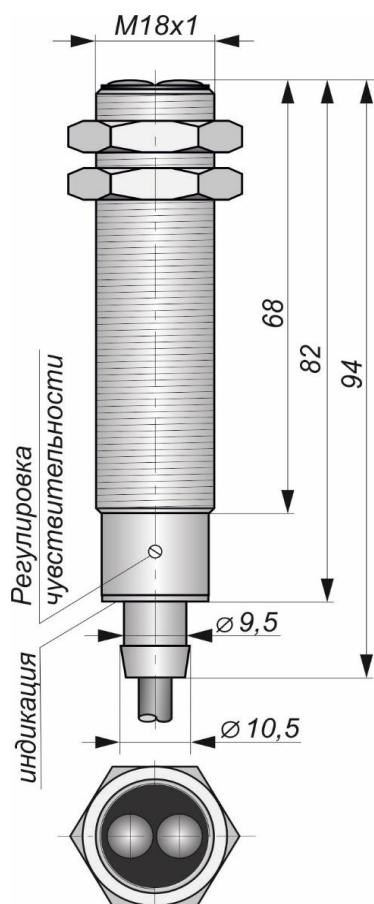
Габаритный чертеж
