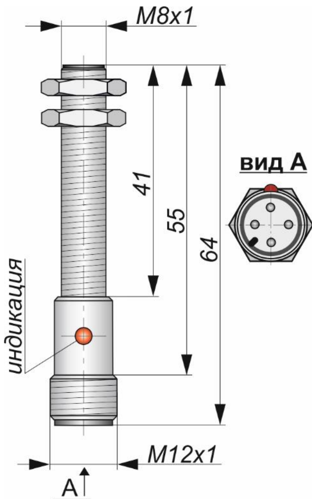
Габаритный чертеж
