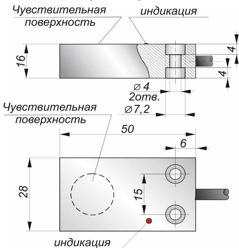
Габаритный чертеж
